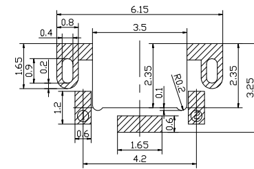
PCB. 焊接图
